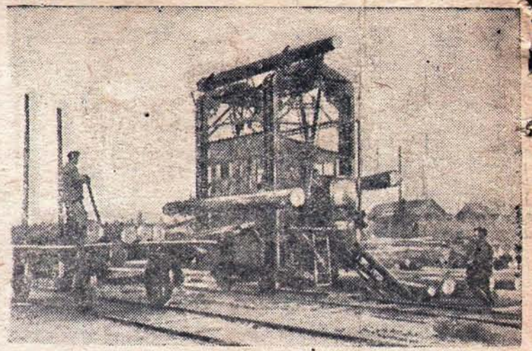
МАРИЙСКАЯ АССР. Коллектив Сулонгерского леспрохоза треста «Марилес» с начала года дал стране сверх плана свыше 30 тысяч кубических метров высококачественной древесины. На снимке: механизированная погрузка леса на железнодорожную платформу элеватором.
