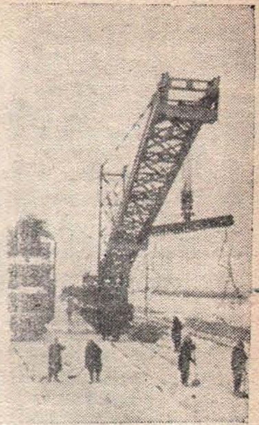
КУЙБЫШЕВСКАЯ ОБЛАСТЬ. На площадку „Куйбышевгидрострой“ со всех концов страны прибывают разнообразные механизмы.
