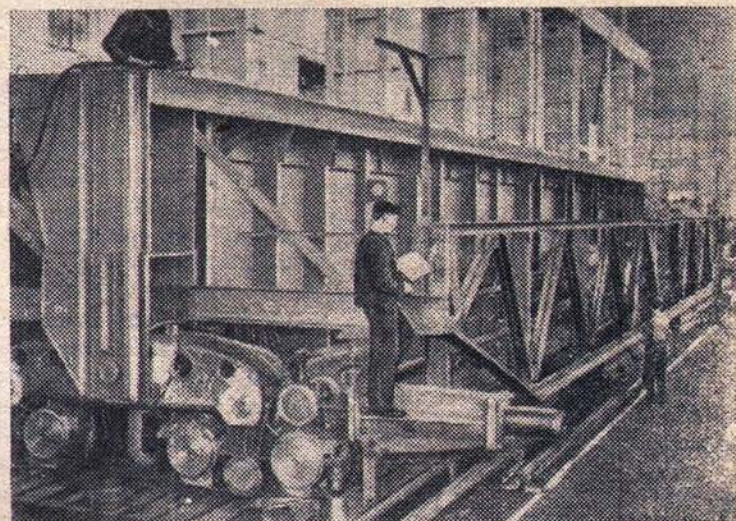
Свердловск. Коллектив Уралмашзавода выпустил новый мощный кран, предназначенный для извлечения стальных слитков из изложниц. Новый кран предназначается для одного из металлургических предприятий Китайской Народной Республики. На снимке: монтаж нового крана.
