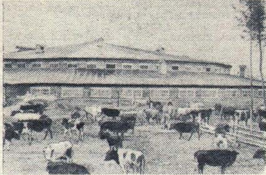
Иркутская область. В колхозе имени Ворошилова Куйтунского района сооружен оригинальный круглый коровник на 400 голов. Диаметр коровника — 54 метра. В его центральной части оборудован профилакторий, где содержатся новорожденные телята. Коровник круглой формы отличается от обычного рядом преимуществ, из которых одно из главных — хорошая обтекаемость, предохраняющая животных от сильных зимних ветров.
