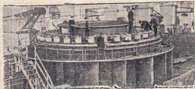
Коллектив Харьковского турбинного завода изготовил гидротурбину для Иркутской ГЭС. На снимке: подготовка турбины к отправке.
