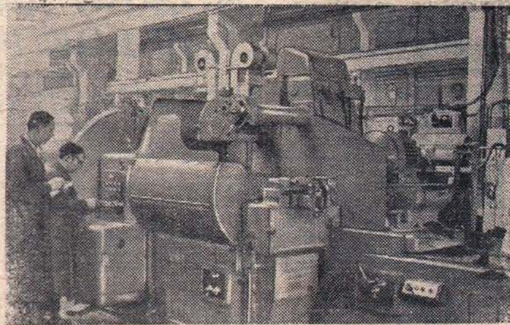
На московском заводе шлифовальных станков изготовлен опытный образец нового зубошлифовального станка модели «5860А». Станок предназначен для шлифования профиля зубьев, термически обработанных зубчатых колес диаметром до 800 миллиметров и наибольшим модулем 12 миллиметров. Станок работает по полуавтоматическому циклу, обеспечивая точность обработки зубьев таких колес с точностью по шагу между зубьями до 0,004—0,005 миллиметра.
